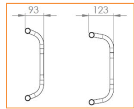
030403 & 030404 Rückenbügel oval eng und weit
